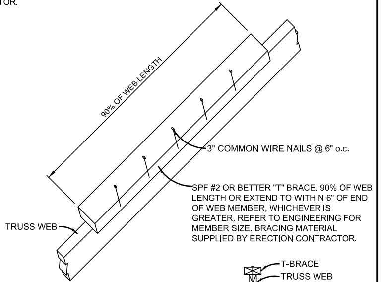
T-BRACE DETAIL
